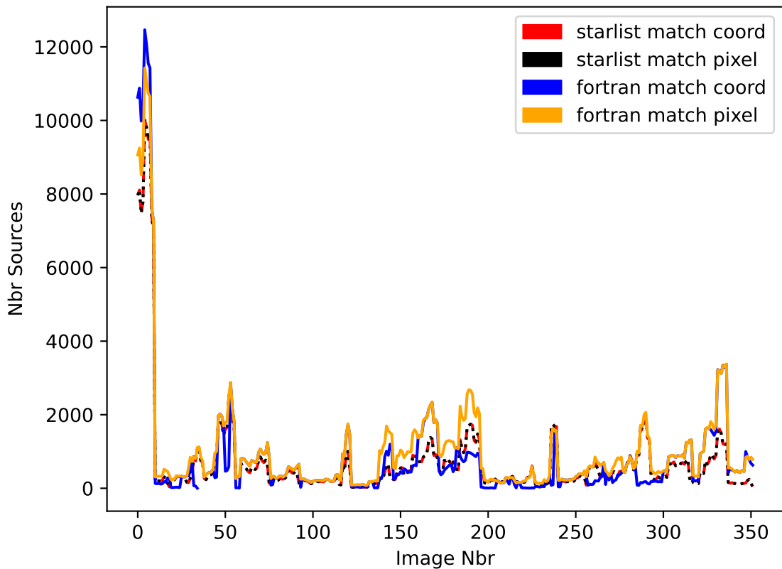
RA/DEC vs Pixel Matching - RA/DEC Ok?
